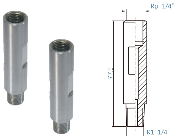
延长杆
